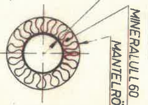
SKORSTENSPÖR SKALA 1:10
